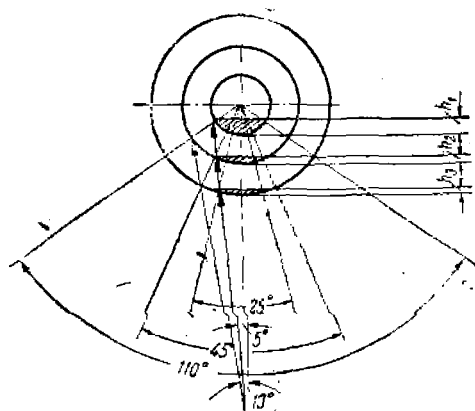
Фиг. 78. Положения копы при различных диаметрах рольки.
