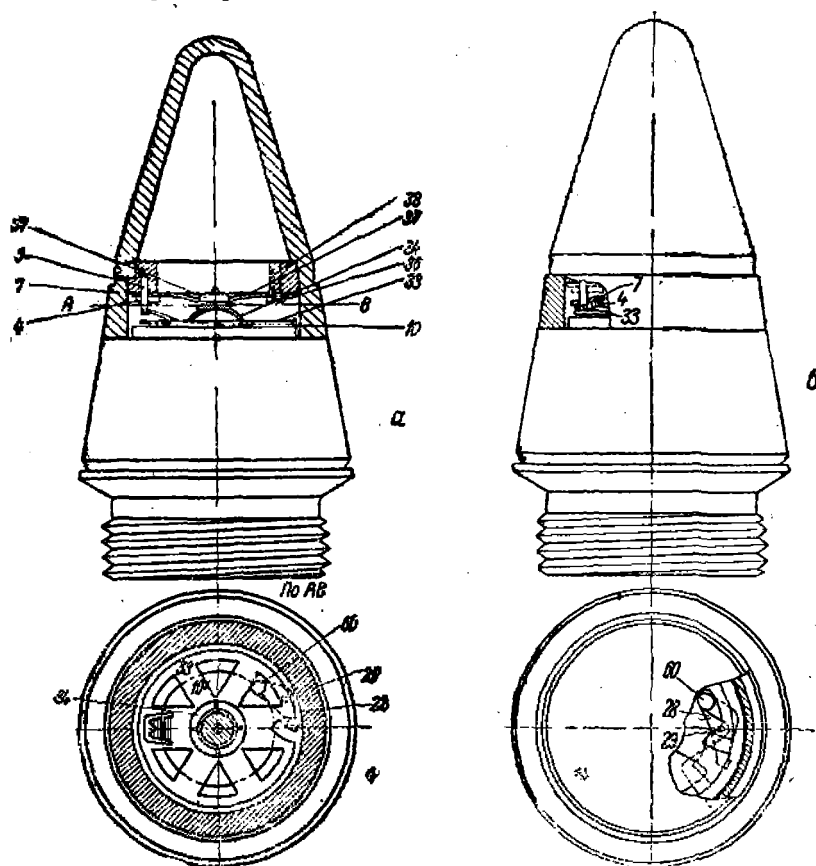
Фиг. 179. Пусковой механизм трубки Юнгана. а — до выстрела; б — после выстрела.
