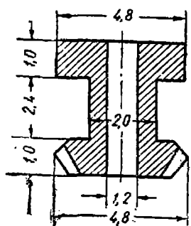
Фиг. 149. Шестерня баланса трубки Варо-
