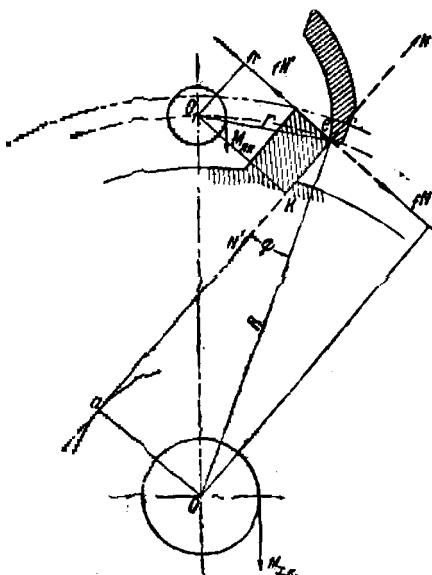
Фиг. 102. Моменты и силы в ходе Юнгаса:
