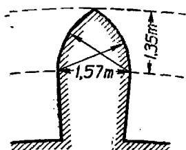
Фиг. 54. , Графическое построение зуба колеса
