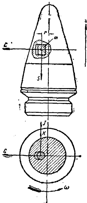
Фиг. 25. Схема сил, действующих на трубку при движении снаряда по каналу орудия.
