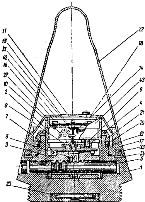
Фиг. 186. Трубка Варо.
