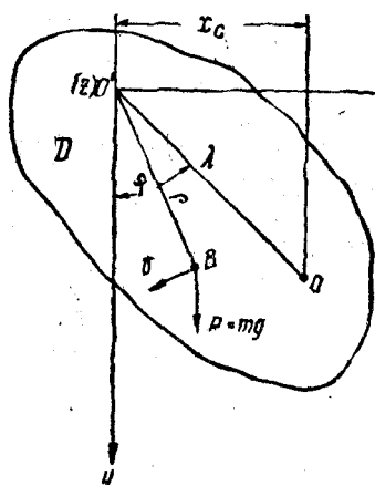
Фиг. 156. Определение периода колебания физического маятника.
