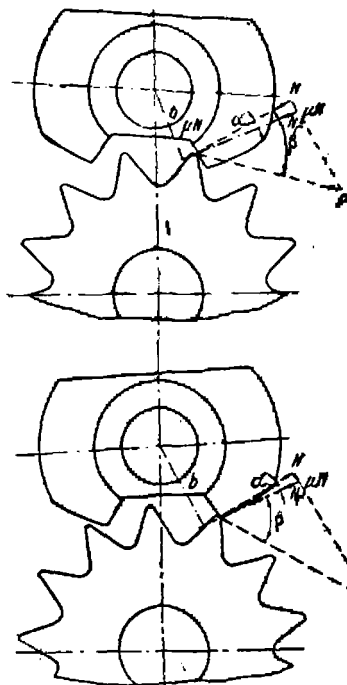
Фиг. 110. Определение крутящего момента на выходной палете:
