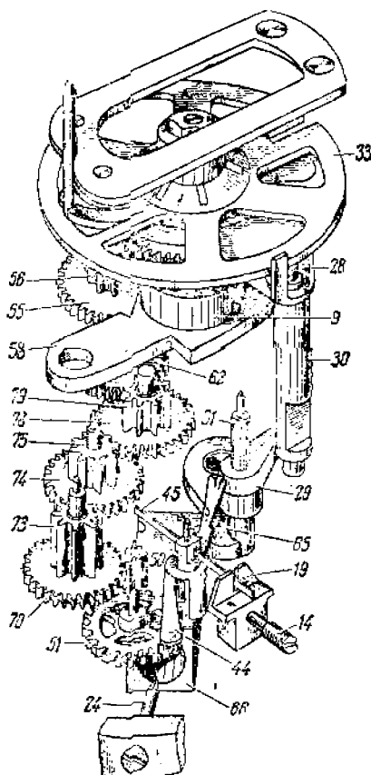
Фиг. 184. Кинематическая схема трубки Юнгана.
