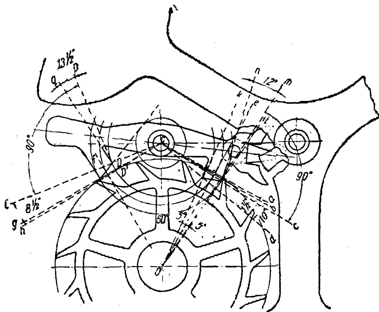
берется несколько больше ширины пальца F , чтобы обеспечить надлежащий зазор между деталями и чтобы язык F не застревал в вырезе вилки во время колебания баланса (зазор берется от 0,02 до 0,03 мм).
