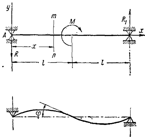
Фиг. 135. Определение упругой линии.
