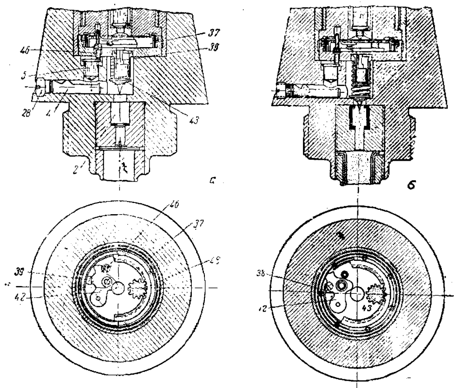
Фиг. 199. Спусковой механизм трубки Варо.
