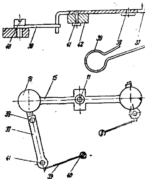
Фиг. 190. Центробежный предохранитель баланса трубки Варо.
