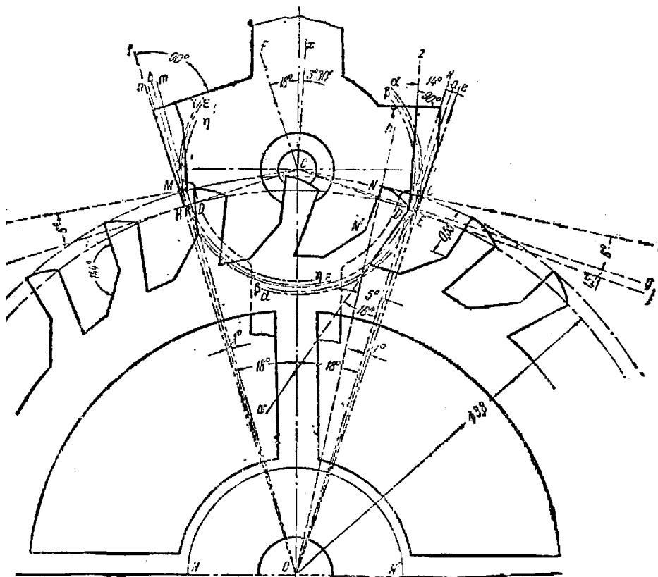
Фиг. 97. Графическое построение неравноплечевого хода Тиль-Круппа.
