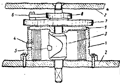
Фиг. 5. Неподвижный барабан часового механизма.
