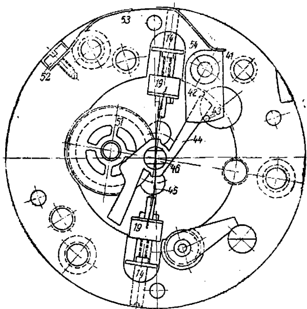
Фиг. 182. Регулятор трубки Юнгаса.
