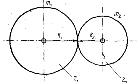
Фиг. 47. Определение модуля по расстоянию между центрами колеса и триба.
