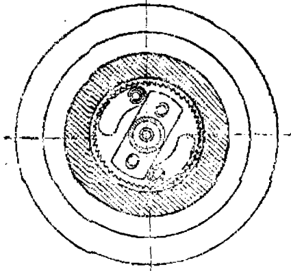
Фиг. 200. Предохранительный и пусковой механизм трубки Варо.
