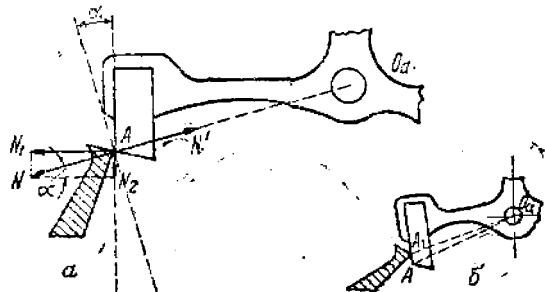
Фиг. 82. Схема действующих сил во время «притяжения».
