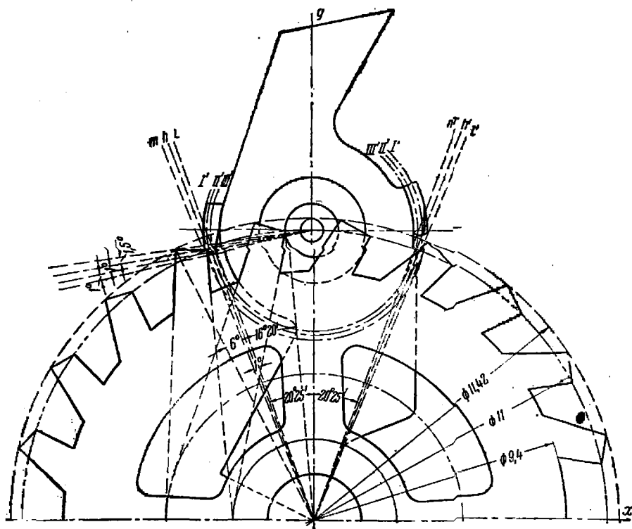
Фиг. 101. Зуб на входной палете хода Юнгса
