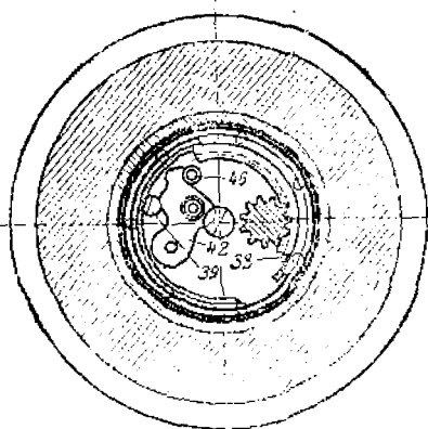
Фиг. 200. Предохранительный и пусковой механизм трубки Варо.
