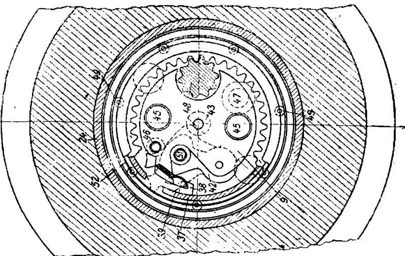
Фиг. 197. Действие установочного механизма трубки Варо.
