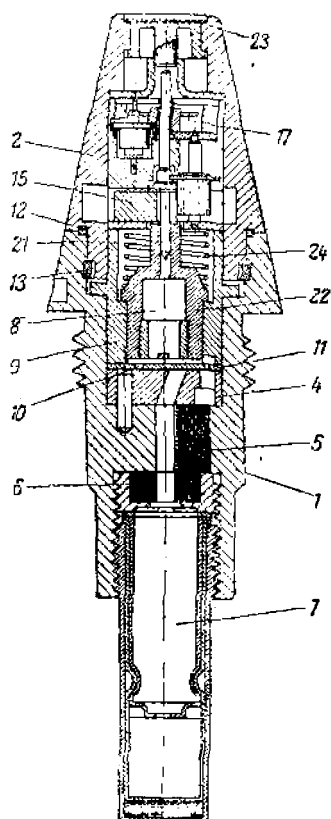
Фиг. 201. Взрыватель Тауро.
