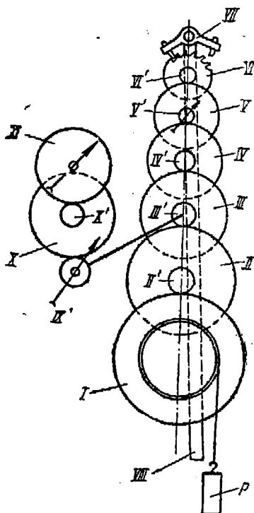
Фиг. 2. Общая схема часового механизма.
