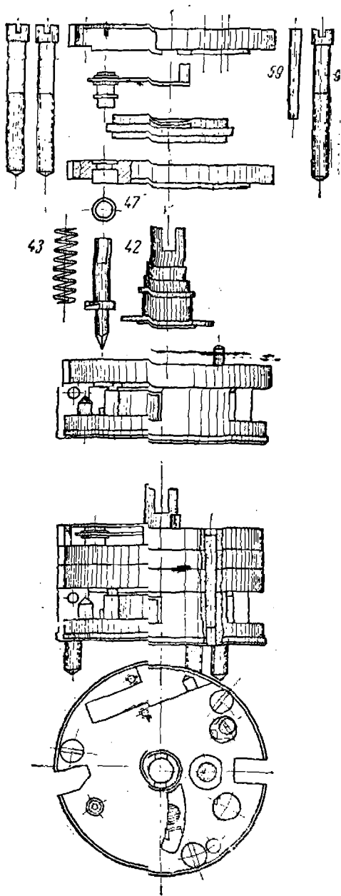
Фиг. 174. Движущий и пусковой механизмы трубки Тиль-Круппа. Схема сборки механизмов.
