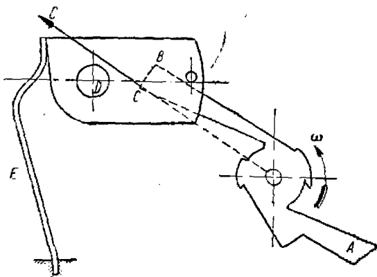
Фиг. 89. Схема баланса и центробежного предохранителя трубки Юнгана.
