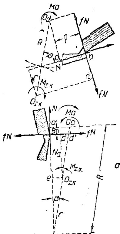
Фиг. 84. Соотношение моментов сил в анкерном ходе.
