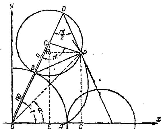
Фиг. 50. Построение эпициклоиды.
