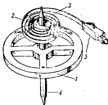
Фиг. 111. Баланс со спиралью 1—баланс; 2—ролька волоска; 3—спираль; 4—ось баланса; 5—коб- лочка баланса;
