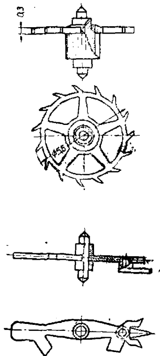
Фиг. 93. Анкерное колесо и вилка трубки Дикси.
