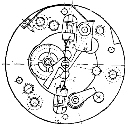
Фиг. 115. Регулятор в трубке Юнгана.
