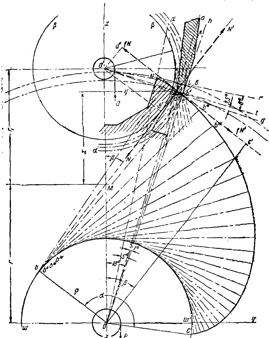
Фиг. 98. Профилирование импульсной поверхности зуба ходового колеса и палеты.
