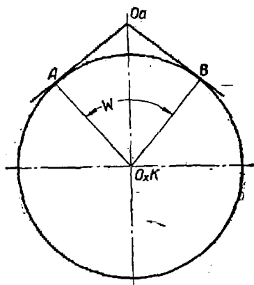
Фиг. 72. Угол обхвата ходового колеса анкером.
