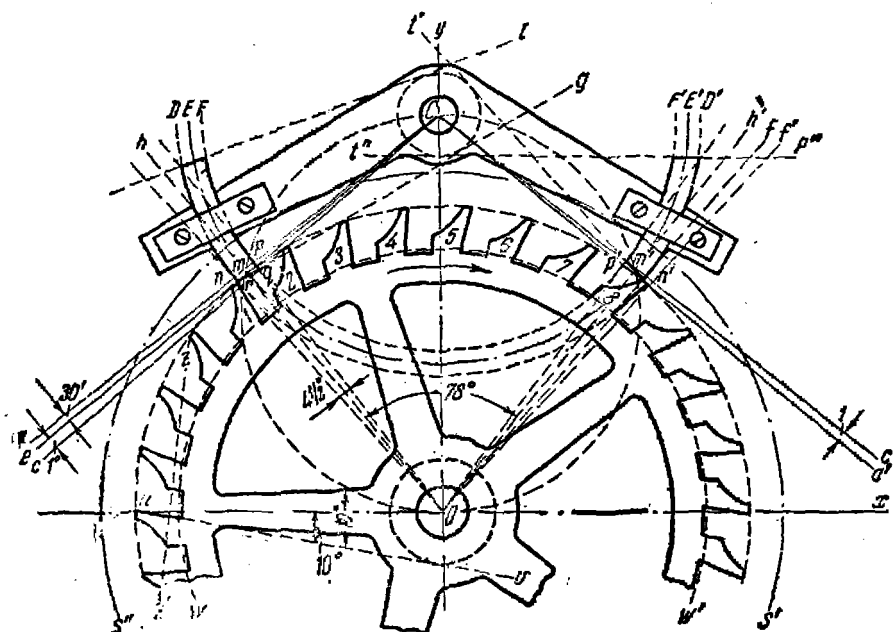
Фиг. 76. Построение хода Грахэма.
