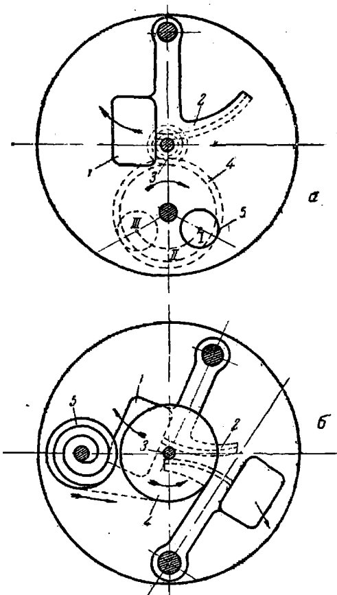
Фиг. 30. Компенсаторы для постоянства момента в двигателе Юнгаса.
