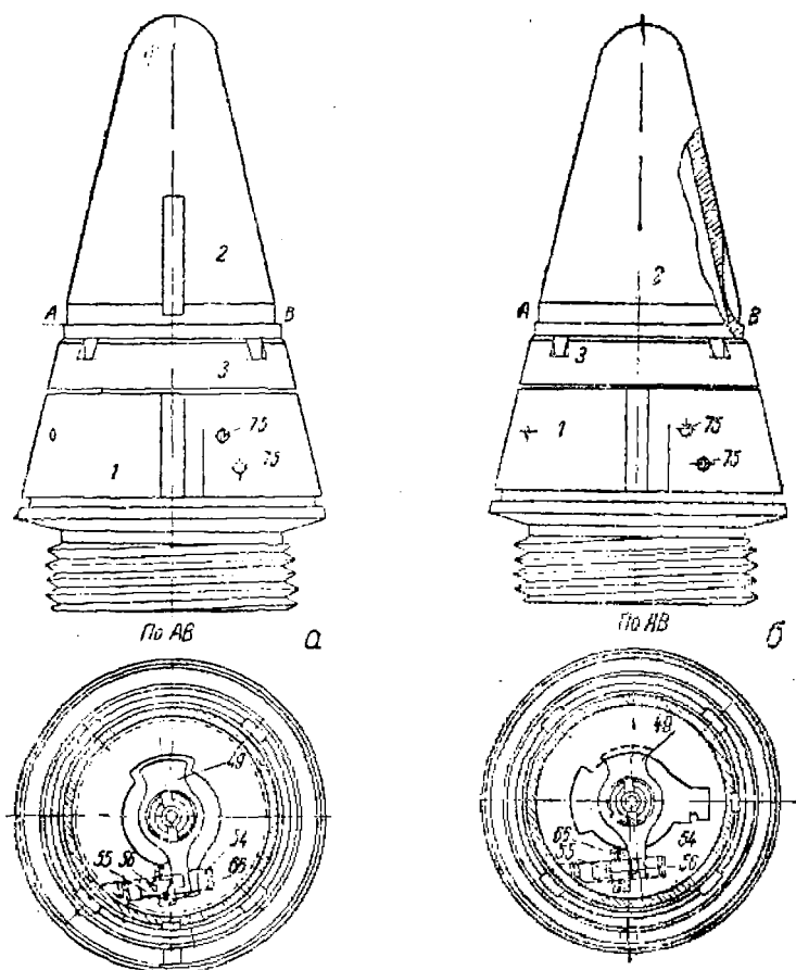
Фиг. 150. Установочный механизм трубки Тиль-Круппа. а—установка на 20 сек.; б—установка на нуль.
