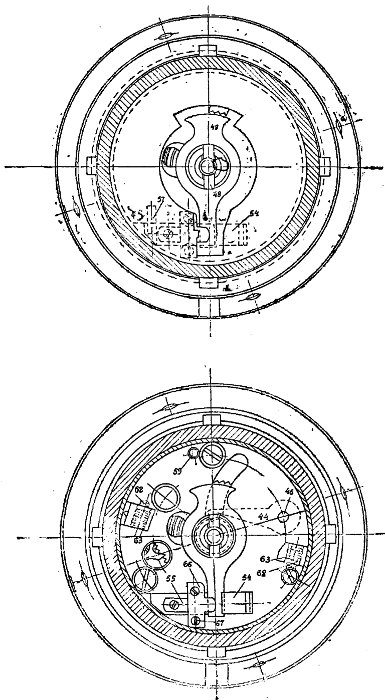
Фиг. 129. Спусковой механизм трубки Тиль-Круппа.
