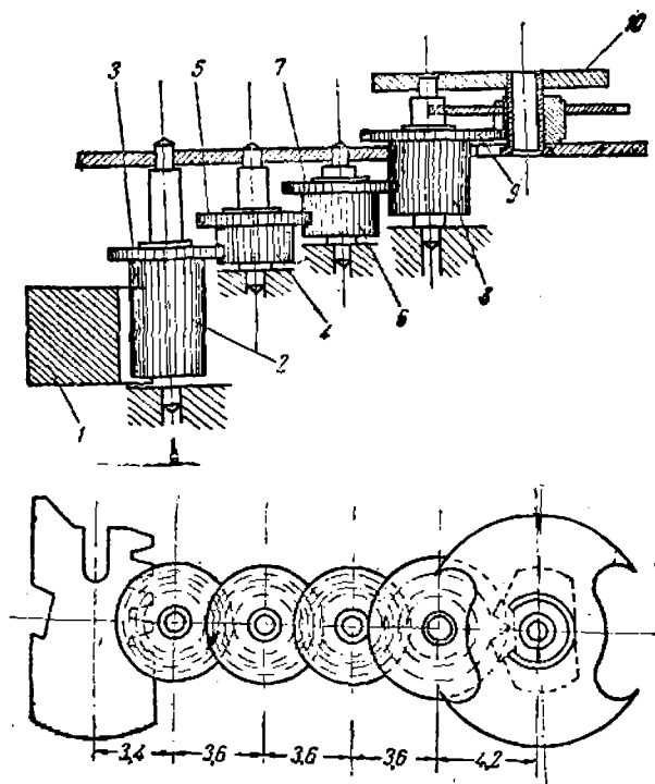
Фиг. 42. Схема часового механизма взрывателя Таваро. 1—кремальера; 2—тр б центрального колеса; 3—центральное колесо; 4—тр б первого промежуточного колеса; 5—первое промежуточное колесо; 6—триб второго промежуточного колеса; 7—второе промежуточное колесо; 8—триб ходового колеса; 9—ходовое колесо; 10—регулятор-баланс.
