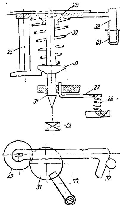
Фиг. 191. Ударный механизм трубки Варо.
