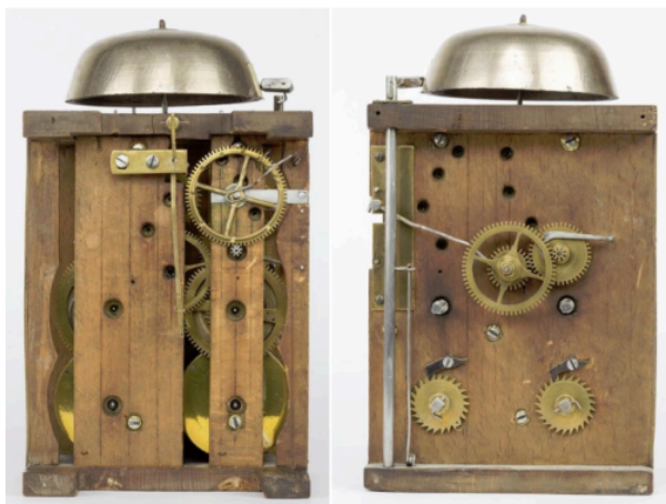
Настольные часы с деревянным механизмом www.heimatmuseumschwarzwald.de Маттиас Хюттлин, Фуртванген
