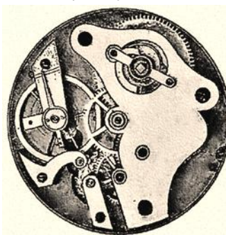
Анкерный спусковой механизм
