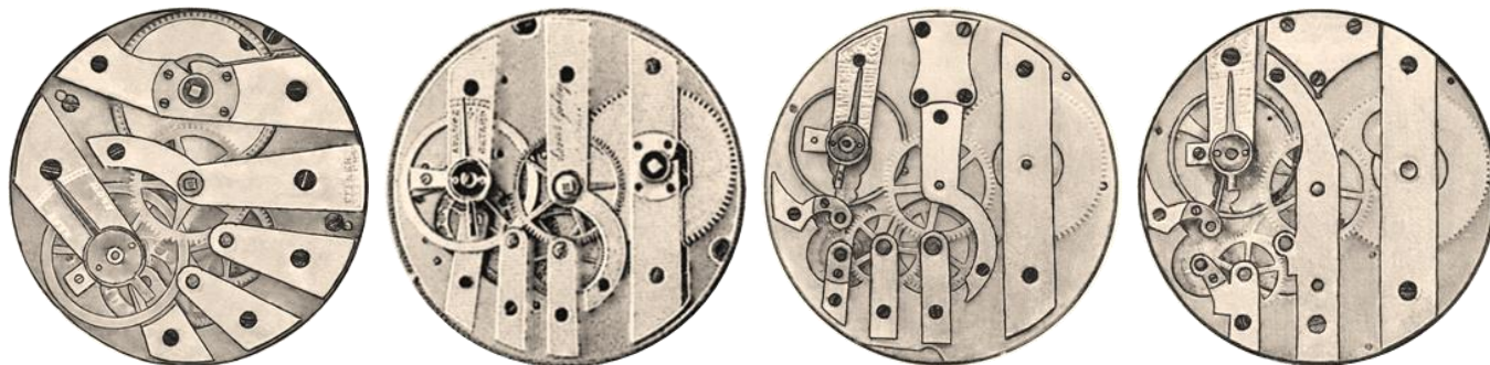
Механизм EPPNER Lepine IV -цилиндр движения со скрипичным ключомиз Женевской школы в 1867 году, затем механизм EPPNER Lepine V с якорным спусковым механизмом и ранним заводом заводной головки и, наконец, соответствующий механизм EPPNER, но теперь с малой секундной стрелкой.
