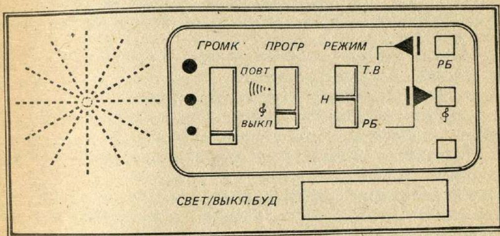
Рис. 34. Органы управления часами 2.14
