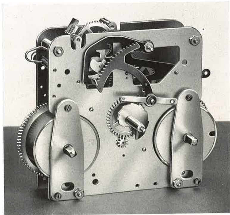
Platinen Plates Platines Platinas 10,8×10,5 cm
