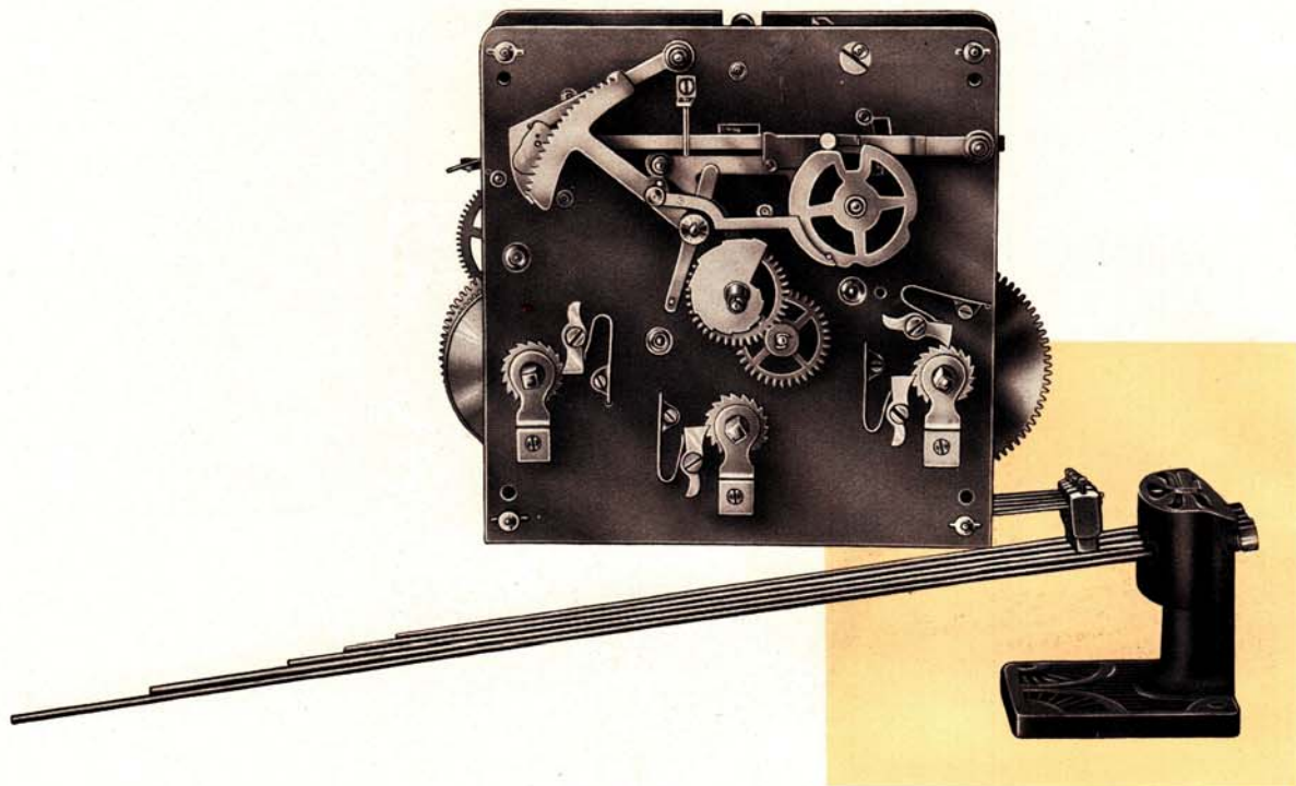
Vorderansicht Front view — Vista delantera — Vue de face
