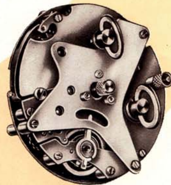
Rückansicht Back view Vista trasera Vue arrière
