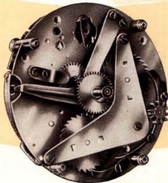
Vorderansicht Front view Vista delantera Vue de face
