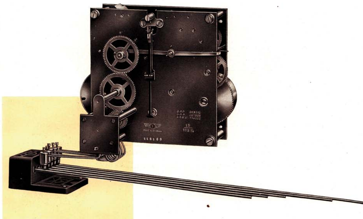
Rückansicht Back view — Vista trasera — Vue arrière
