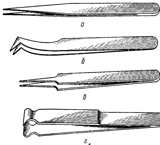
Рис. 11. Пинцеты: а — для работ с деталями часов; б — для установки колес в часовой механизм; в — для работы с волоском; г — для откусывания проволоки
