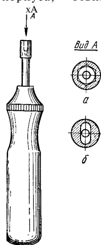
Рис. 37. Ключ для отвертывания гаек и винтов:
