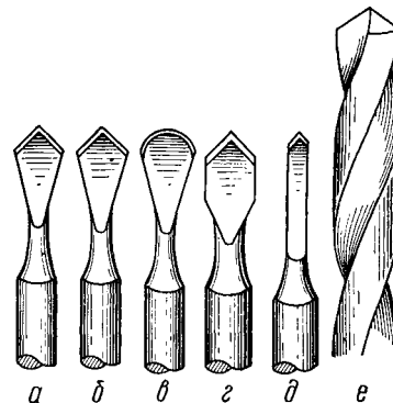
Рис. 21. Перовые сверла: а — одностороннее; б — двустороннее; в — для сверления особо жестких металлов; г — для сверления коротких точных отверстий; д — для сверления мягких металлов; е — спиральное
