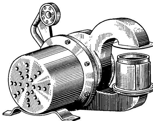
Рис. 93. Сушильный аппарат
