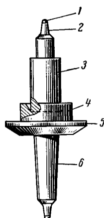
Рис. 68. Ось баланса:
