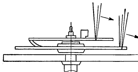
Рис. 104. Исправление плоскости волоска пинцетом
