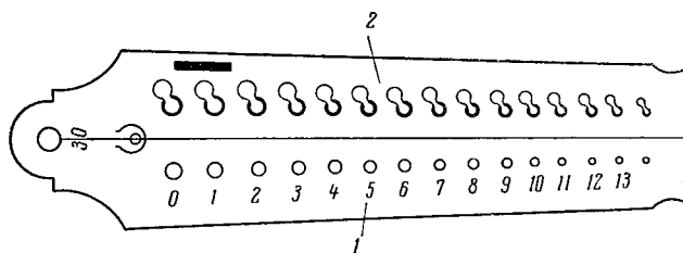
Рис. 15. Винторезная доска:
