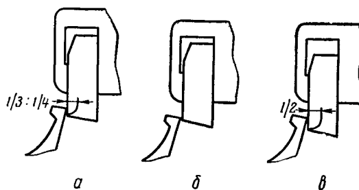
Рис. 97. Угол покоя:
