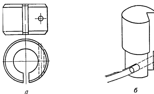
Рис. 71. Колодка и колонка волоска:
