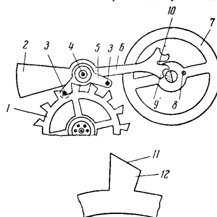
Рис. 46. Спускной механизм будильника*
