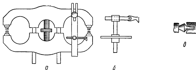
Рис. 83. Лауфциркуль для правки оси баланса:
