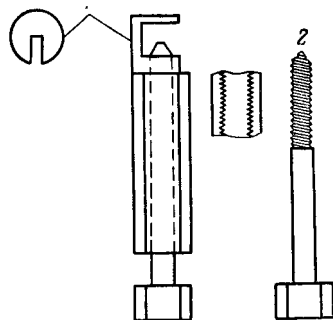
Рис. 81. Приспособление для съема двойного ролика: 1 — патрон; 2 — выталкиватель
