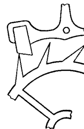
Рис. 65. Английский спуск
