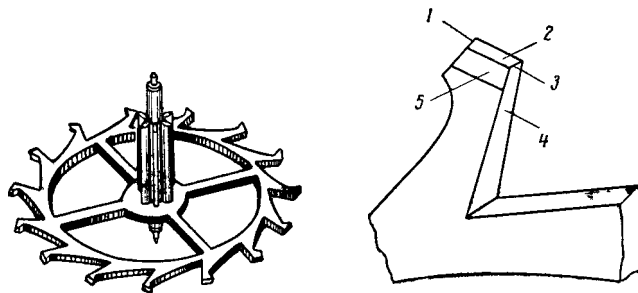
Рис. 61. Ходовое колесо и элементы его зубьев:
