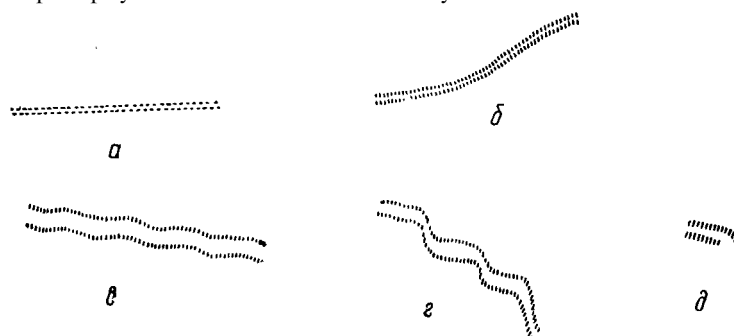
Рис. 108. Записи характеристик неисправностей механизма
