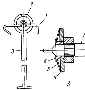
Рис. 36. Скобочный спуск:
