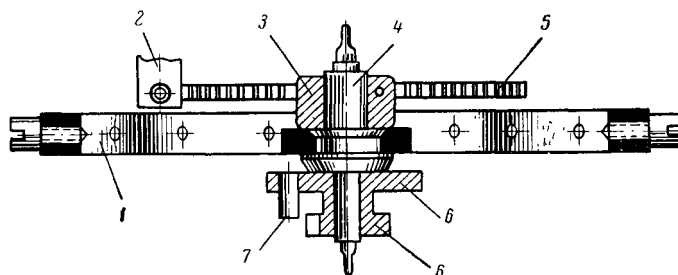
Рис. 66. Спусковой регулятор:
