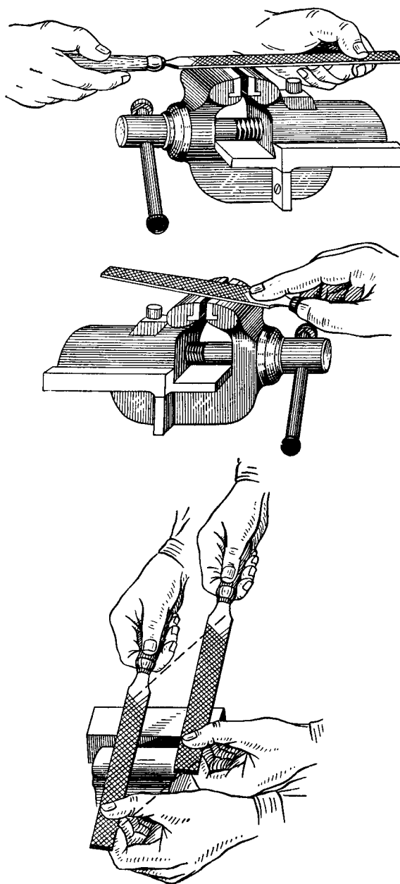
Рис. 18. Правильное положение рук при работе напильником
