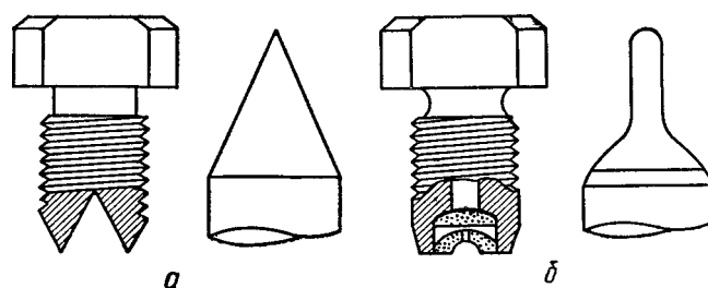
Рис. 52. Центровые винты будильника и формы осей:
