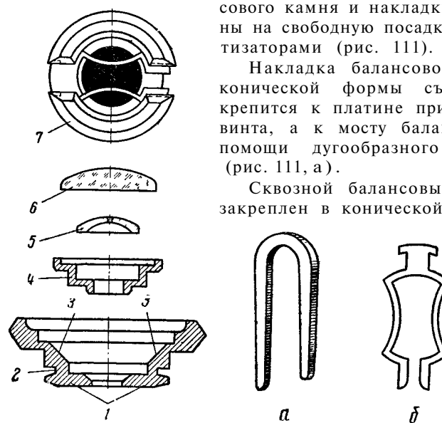
Рис. 111. Детали амортизатора:
