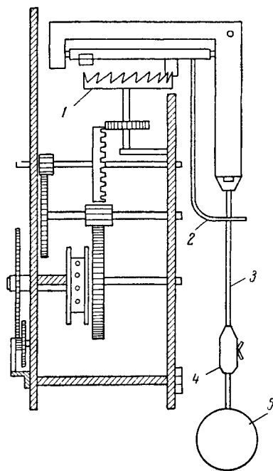
Рис. 5. Шпиндельные часы Гюйгенса:
