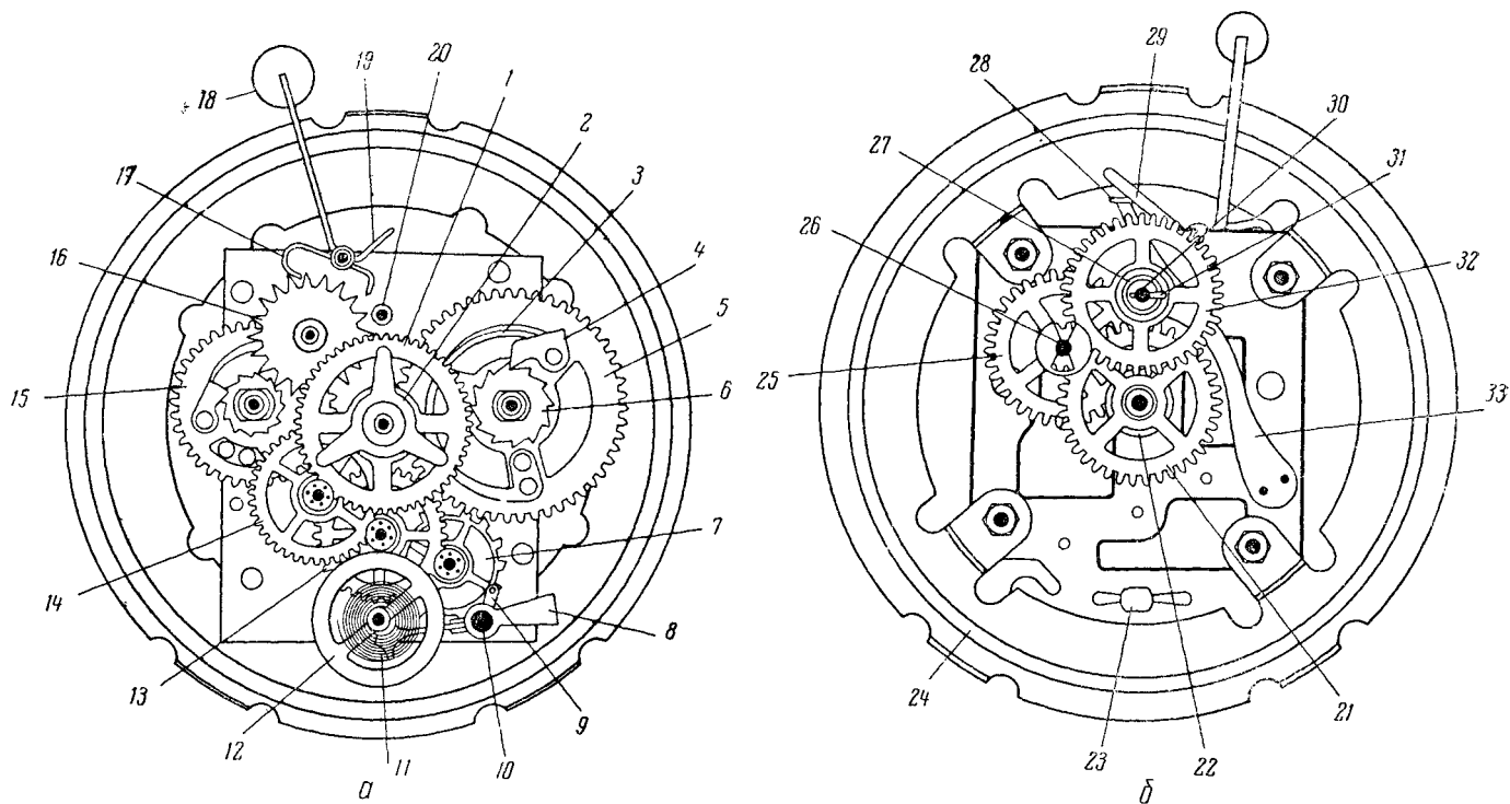
Рис. 44. Механизмы будильника:
