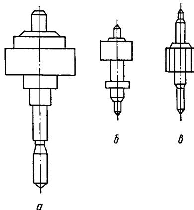
Рис. 60. Трибы колес:
