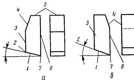
Рис. 63. Палеты:
