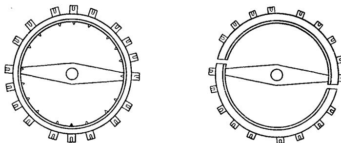
Рис. 67. Балансы:
