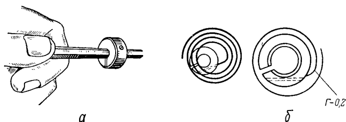
Рис. 87. Заштифтовка волоска:
