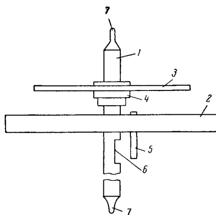
Рис. 47. Узел баланса: 1 — ось баланса; 2 — обод баланса; 3 — волосок; 4 — колодка волоска; 5 — импульсный штифт; 6 — паз оси; 7 — цапфы
