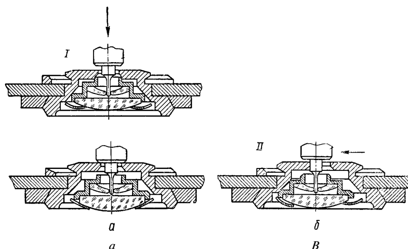
Рис. 112. Работа амортизационного устройства:
