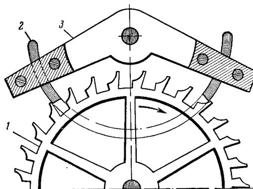
Рис. 6. Крючковый спуск Грахама:
