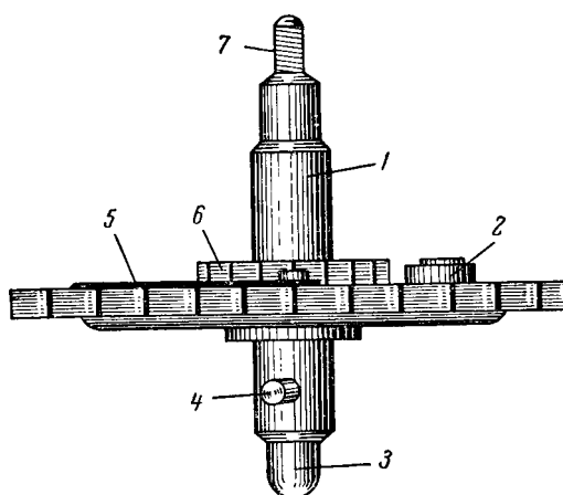
Рис. 45. Заводное колесо:
