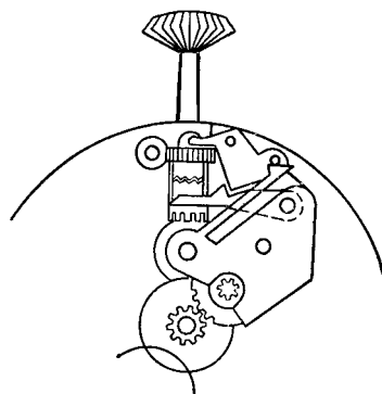
рис. 94. Механизм ремонтара часов КЧ-43
