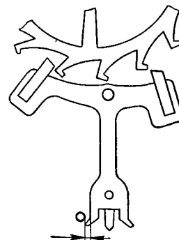
Рис. 100. Потерянный путь
