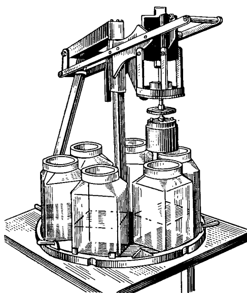
Рис. 92. Моечная машина
