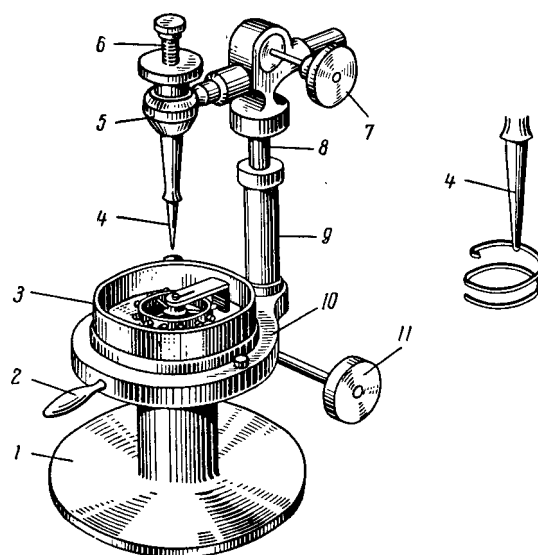
Рис. 88. Вибрационная машинка:
