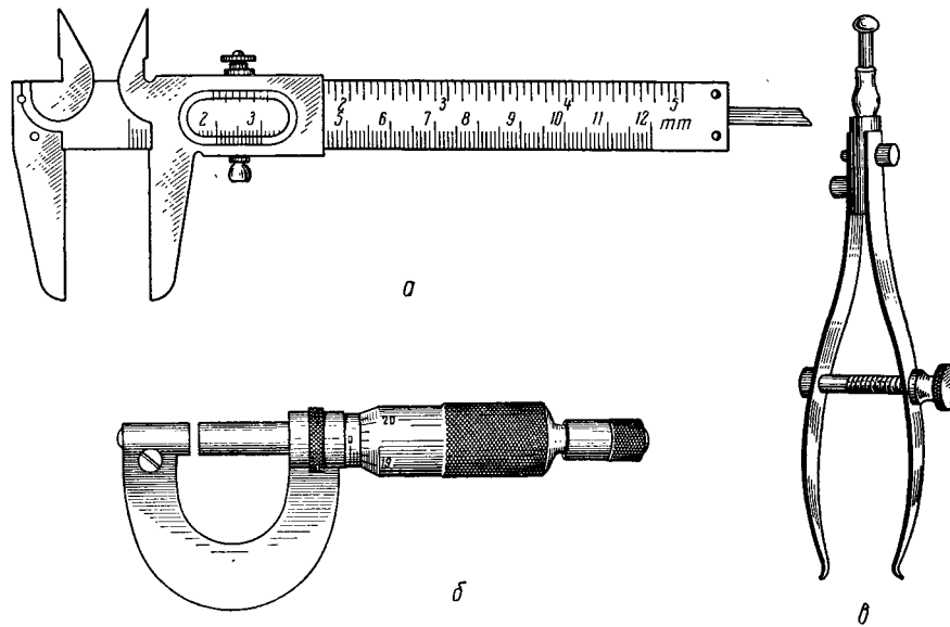
Рис. 17. Мерительные инструменты:
