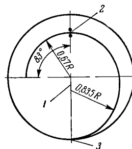
Рис. 90. Форма концевой Беге
