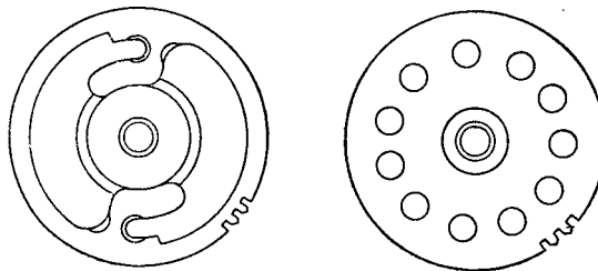
Рис. 50. Заводное колесо
