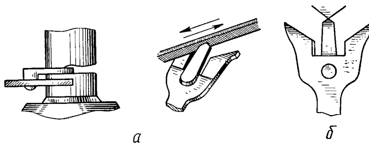
РИС. 102. Регулирование размера копия:
