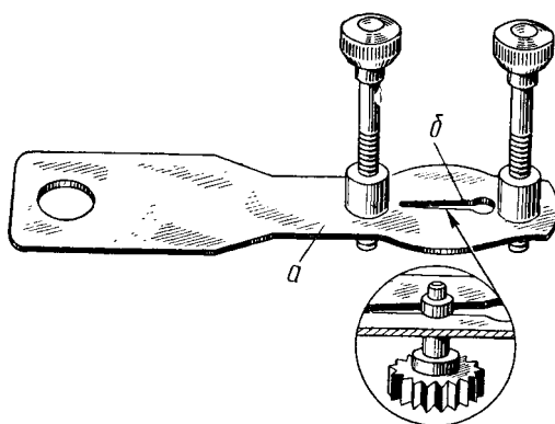
Рис. 78. Приспособление для съема триба а — пластинка; б — прорезь
