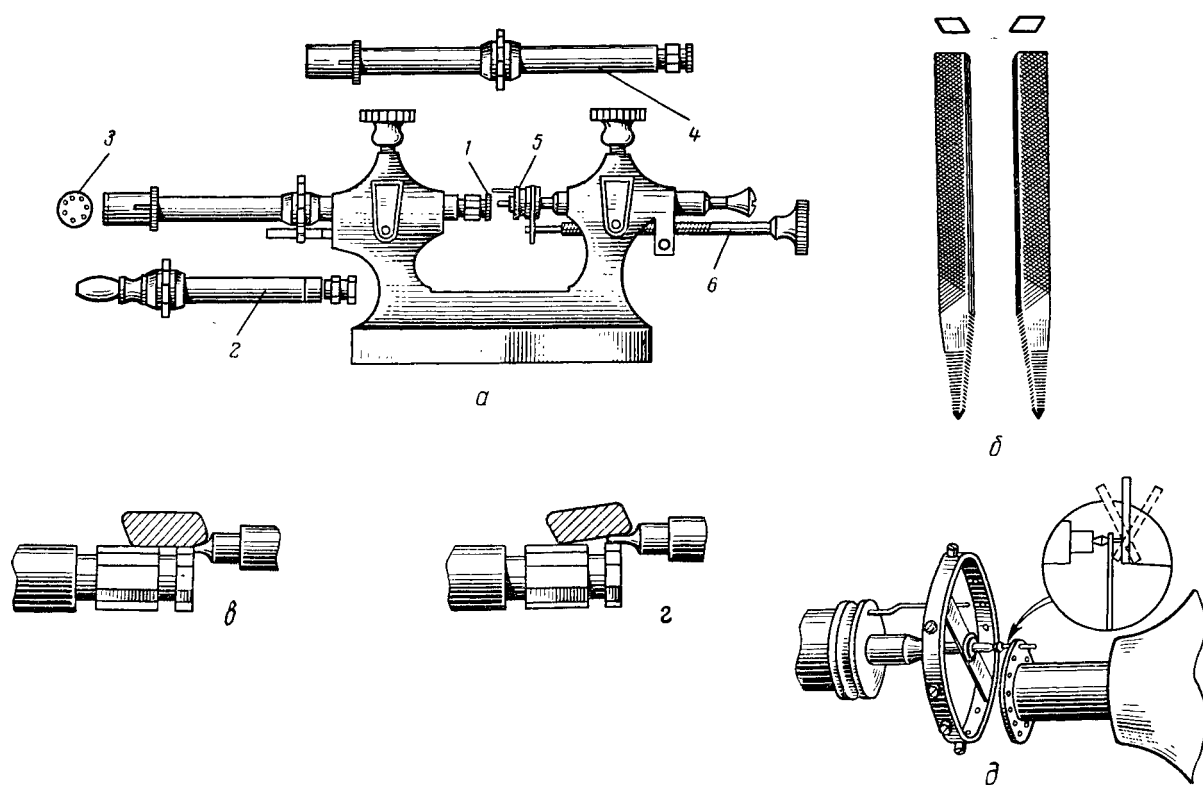
Рис. 86. Схема станка для полирования цапф оси и колес и процесс полирования: а — станок для полирования цапф; б — воронил (полировальники); в — правильное положение полировальника; г — неправильное положение; д — полирование пятки оси / — спица с канавками для полирования цапф; 2 — спица для полирования удлиненных цапф; 3 — спица для полирования пяток; 4 — спица для полирования цапф средней величины; 5 — ролик; 6 — винт
