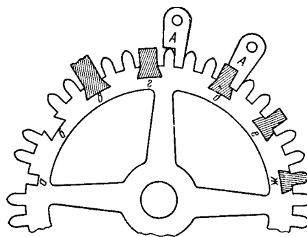
Рис. 40. Последовательность вставки зуба в обод колеса:
