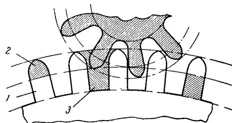
Рис. 32. Элементы зуба колеса: 1 — ножка; 2 — головка; 3 — выядина
