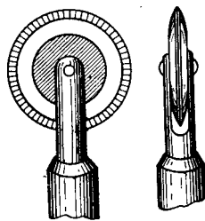
Рис. 39. Роликовый зенкер
