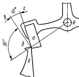
Рис. 99. Угол притяжки
