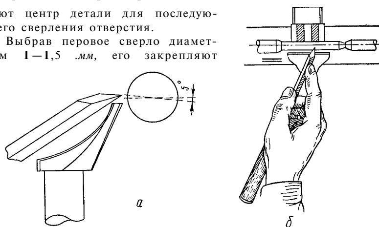
Рис. 27. Работа резцом с подручником:
