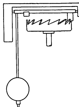
Рис. 4. Шпindelный спуск
